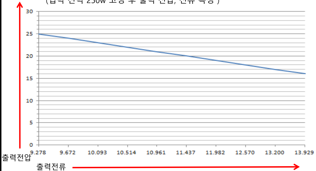
4-2 출력전압-출력전류 그래프 (입력 전력 250w 고정 후 출력 전압, 전류 측정)
