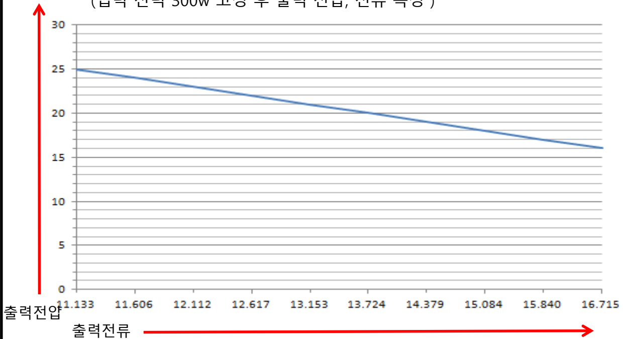
4-2 출력전압-출력전류 그래프 (입력 전력 300w 고정 후 출력 전압, 전류 측정)
