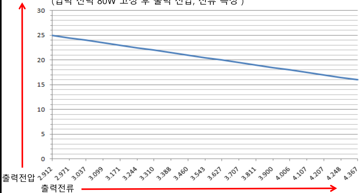
4-2 출력전압-출력전류 그래프 (입력 전력 80W 고정 후 출력 전압, 전류 측정)
