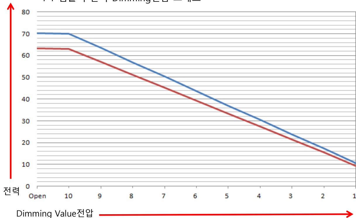
4-1 입출력 전력-Dimming전압 그래프
