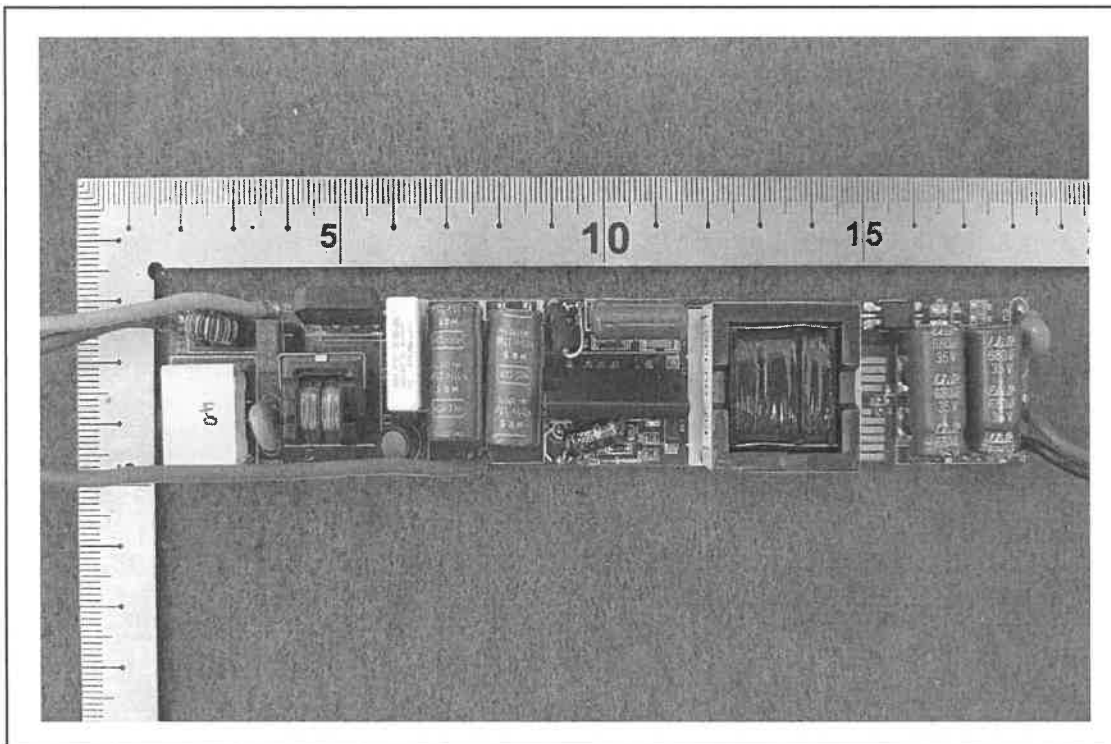
No.4 내부사진(전면)
