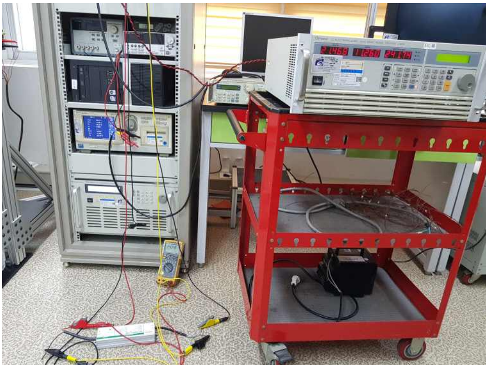
그림 2. 시험 측정 사진
