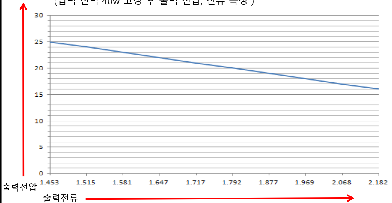
4-2 출력전압-출력전류 그래프 (입력 전력 40w 고정 후 출력 전압, 전류 측정)
