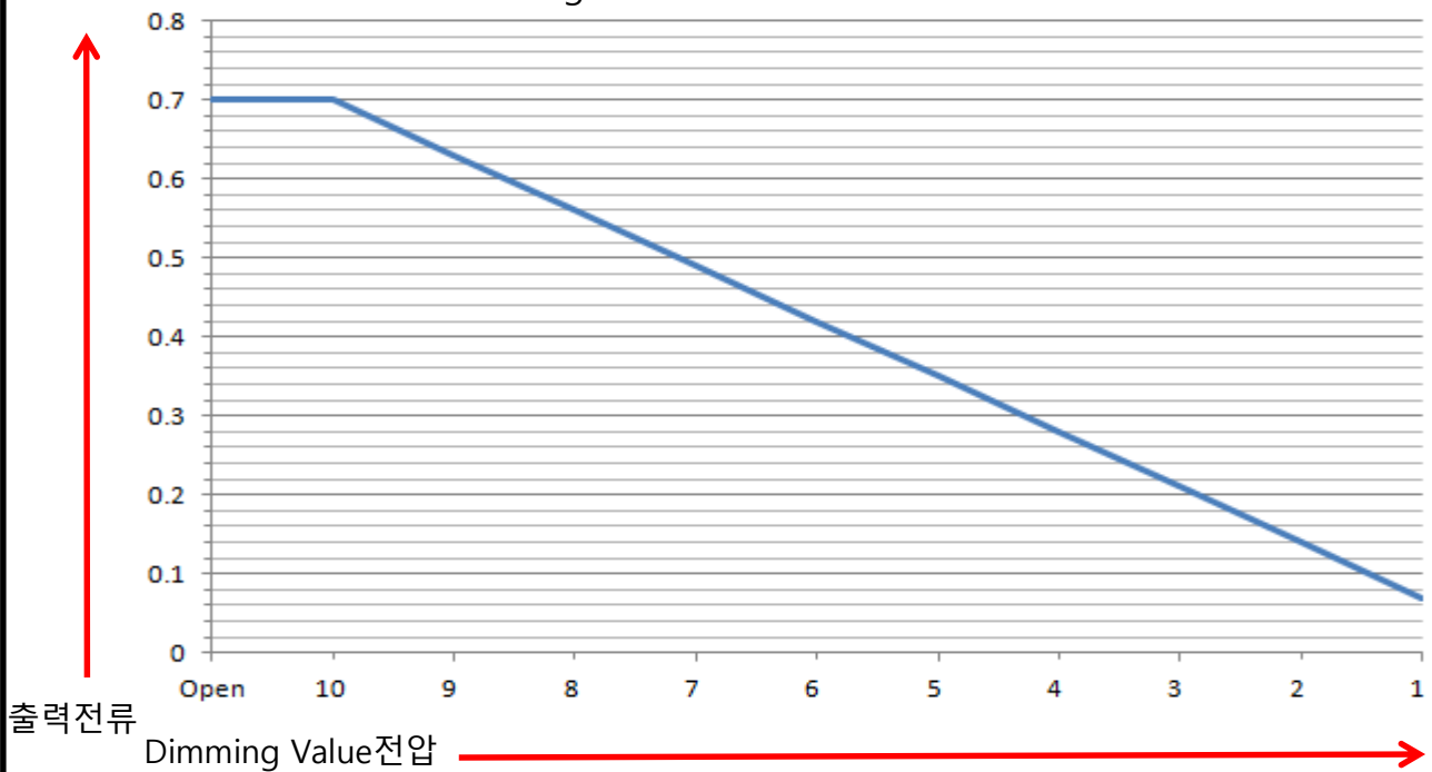
4-2 출력 전류-Dimming전압 그래프
