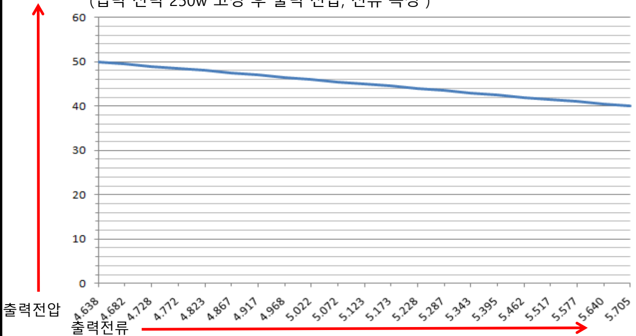
4-2 출력전압-출력전류 그래프 (입력 전력 250w 고정 후 출력 전압, 전류 측정)
