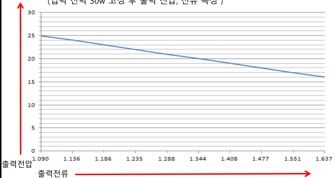
4-2 출력전압-출력전류 그래프 (입력 전력 30w 고정 후 출력 전압, 전류 측정)
