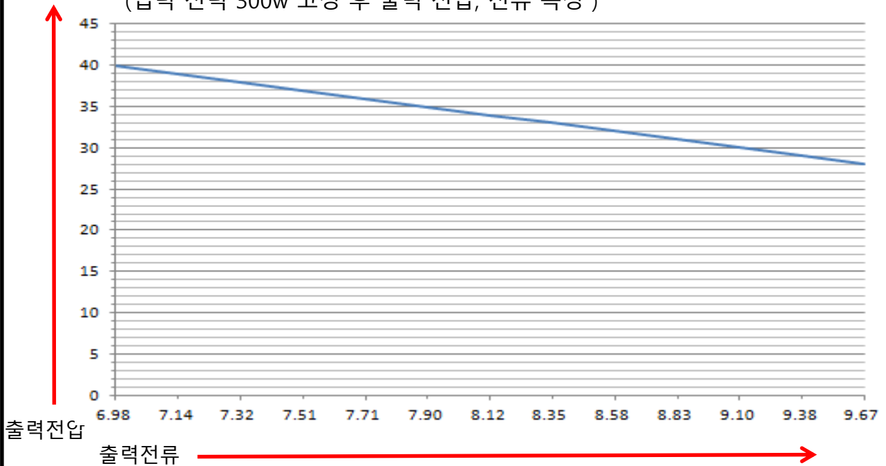
4-2 출력전압-출력전류 그래프 (입력 전력 300w 고정 후 출력 전압, 전류 측정)
