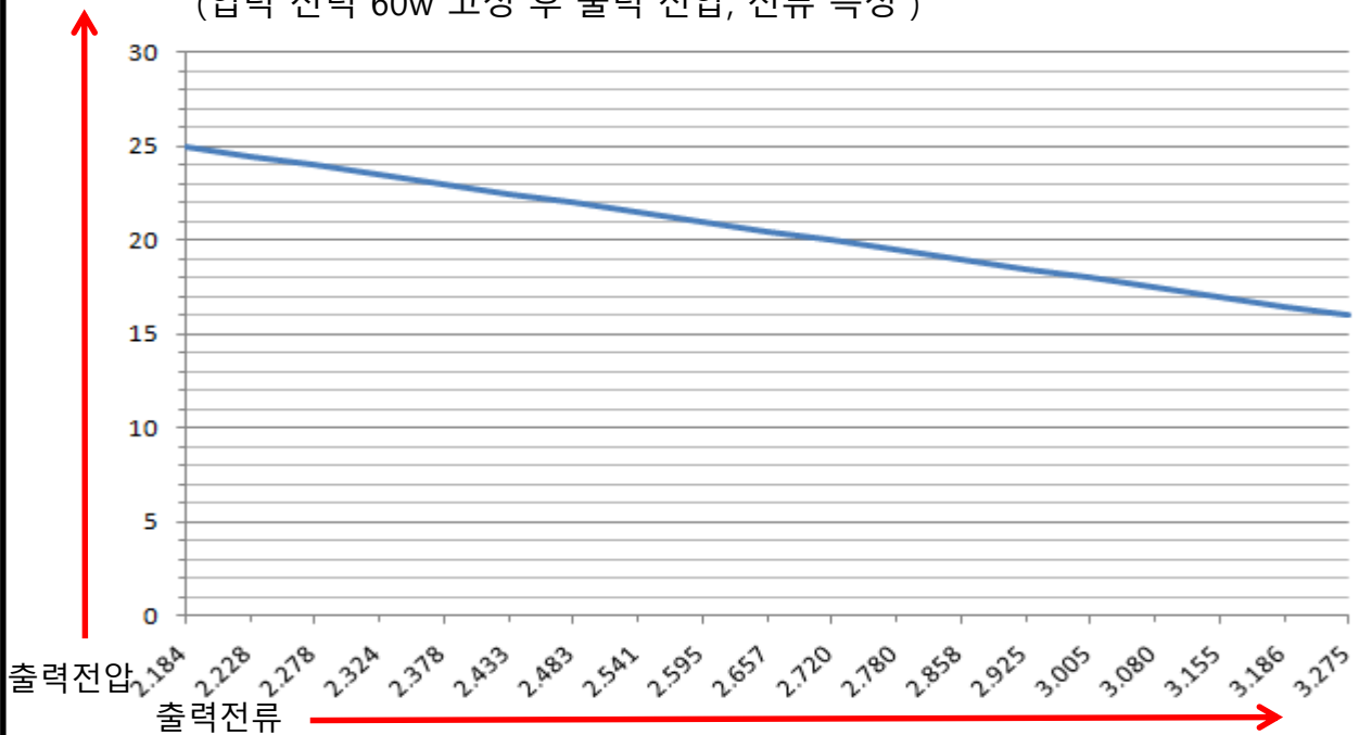
4-2 출력전압-출력전류 그래프 (입력 전력 60w 고정 후 출력 전압, 전류 측정)
