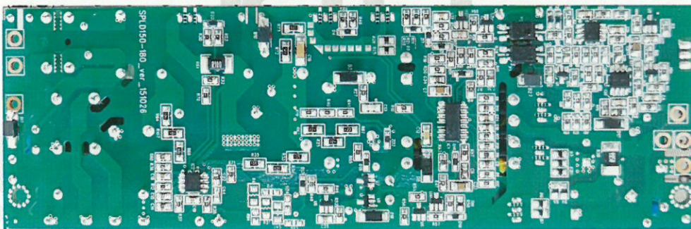
[PCB - 후면]
