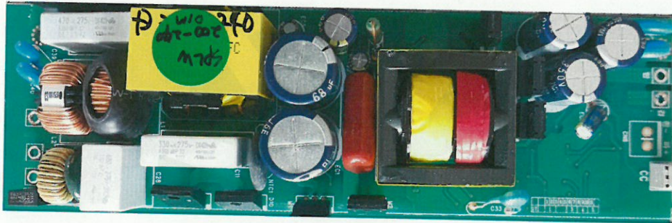
[PCB - 전면]
